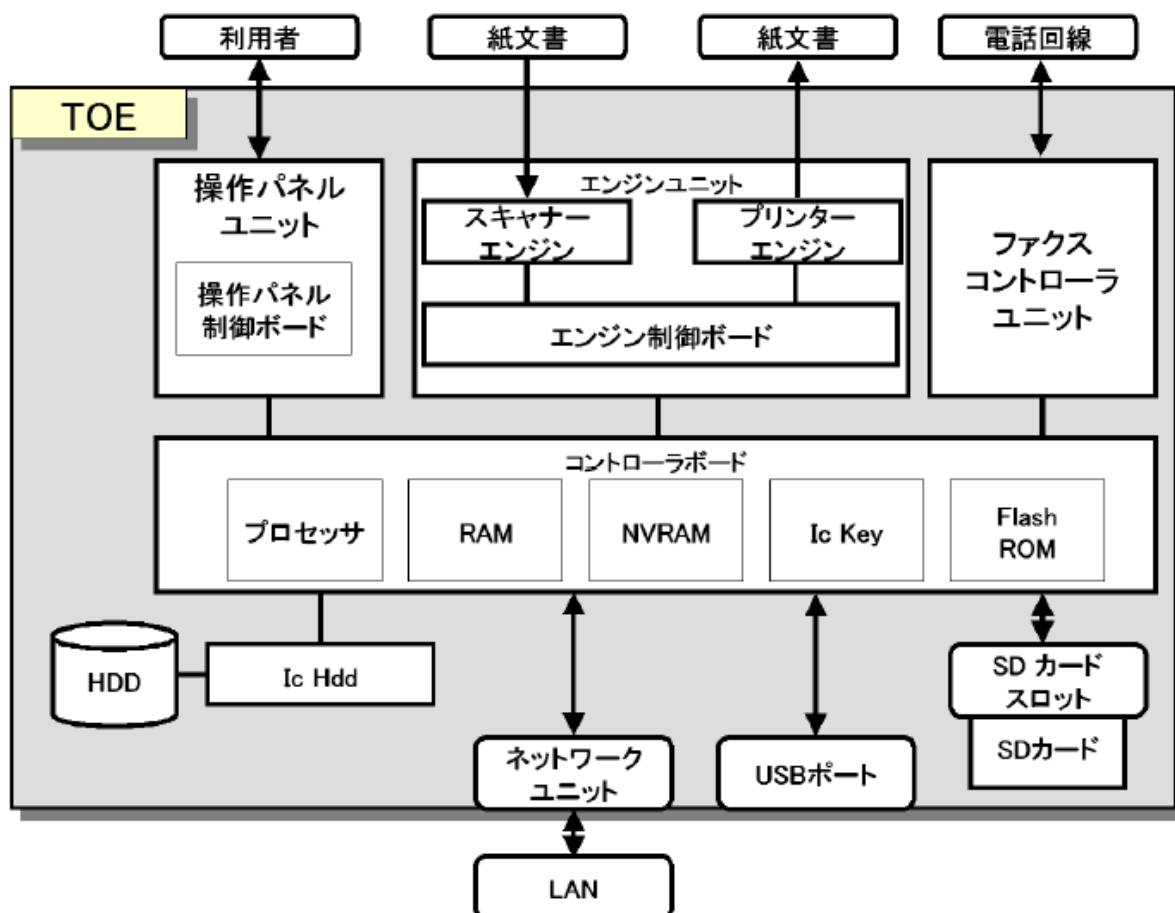
図5-1 TOE境界
