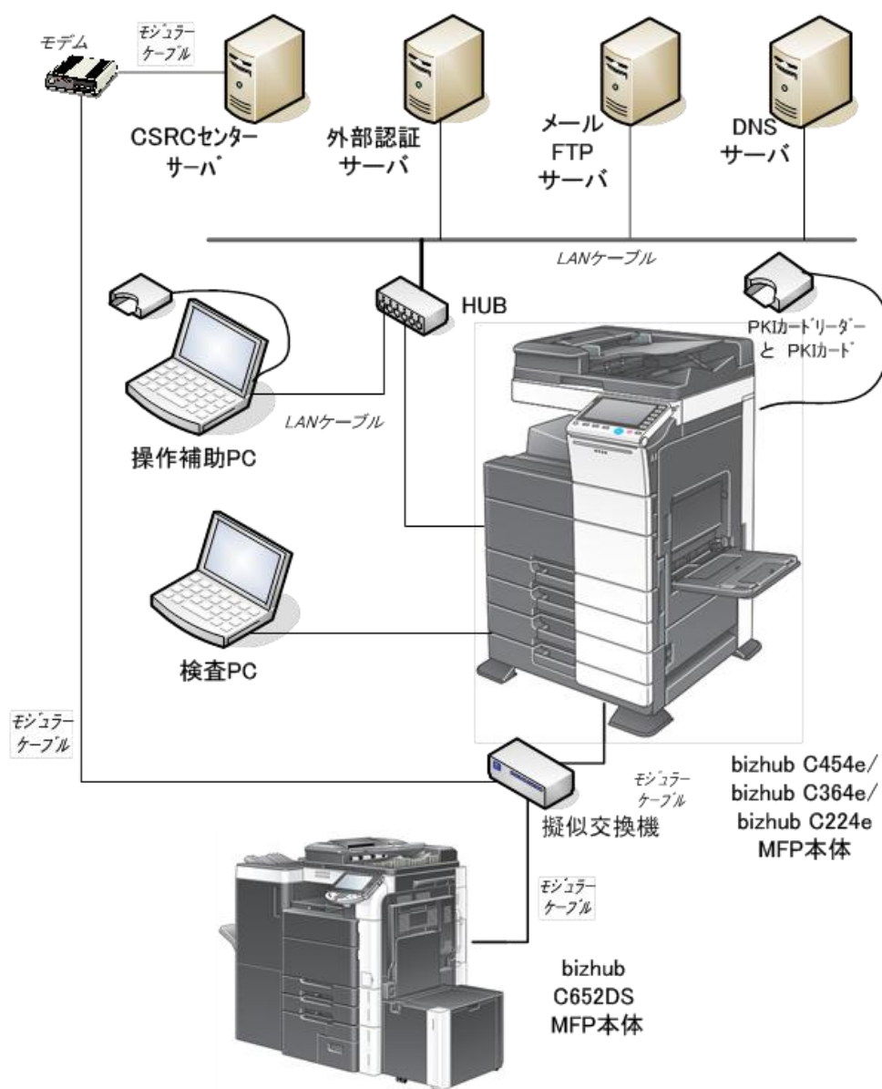
図7-2 侵入テスト環境
