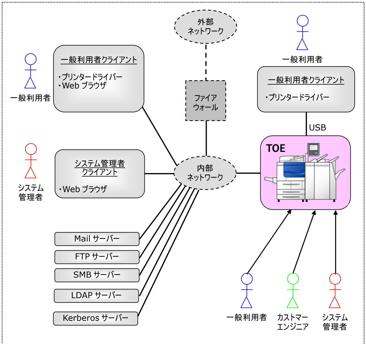
図 1 TOE の想定する利用環境
