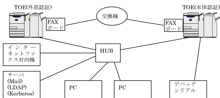
図7-2 独立テストの構成図
