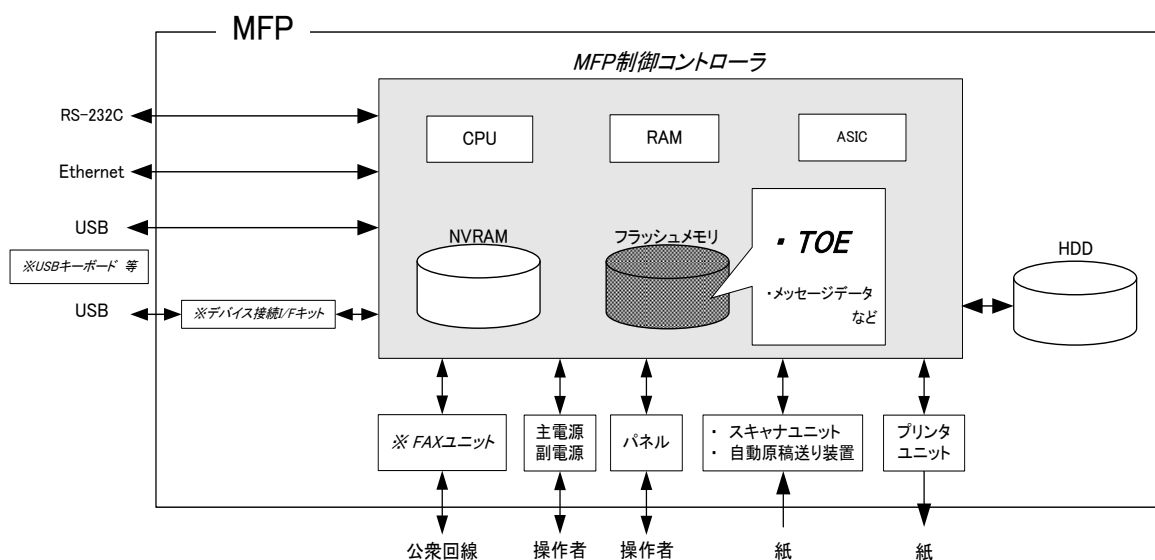
図5-1 TOEに関するハードウェア構成
