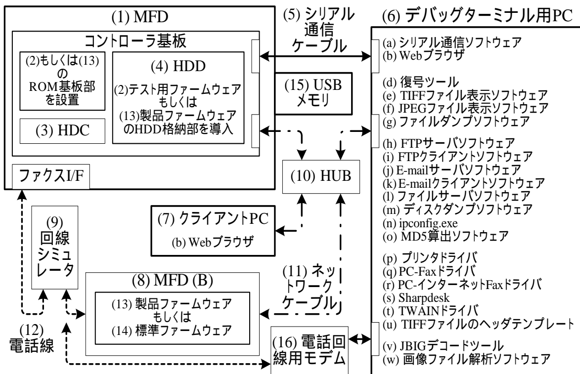
図 7-1 開発者テストの構成図
