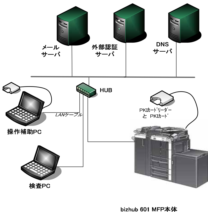
図3-2 侵入テストの構成図
