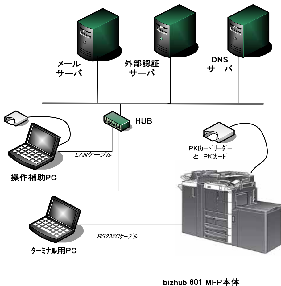
図3-1 開発者テストの構成図
