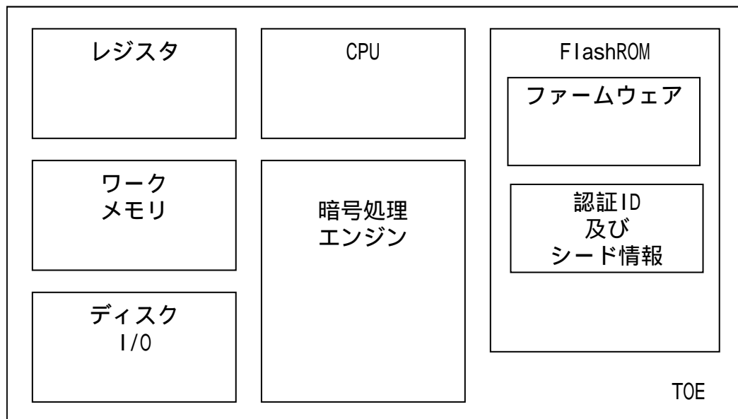
図1-1 TOE物理構成図
