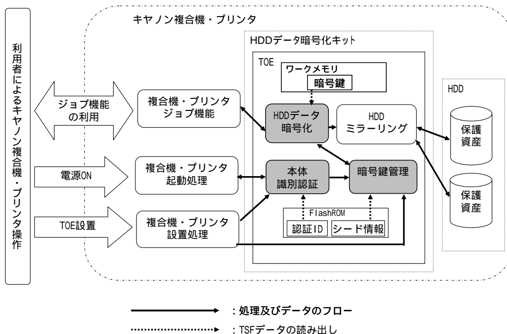
図1-2 TOEの動作概要
