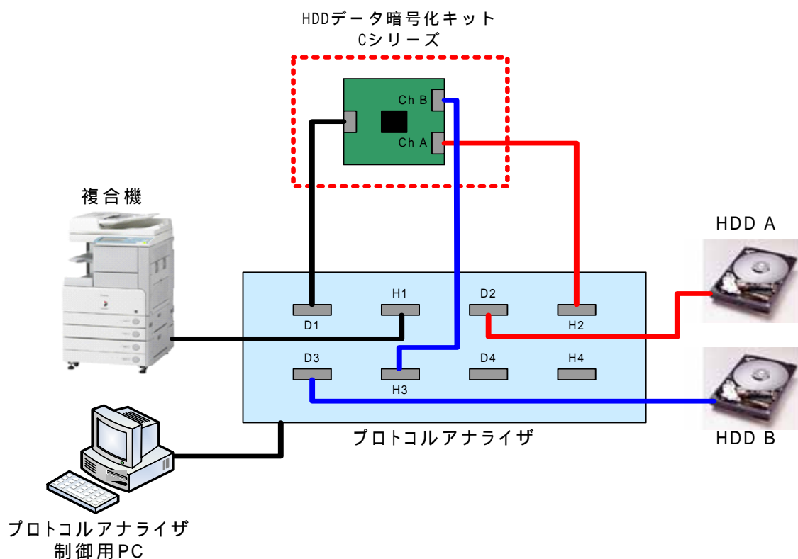
図2-1 開発者テストの構成図(複合機レベルテスト)
