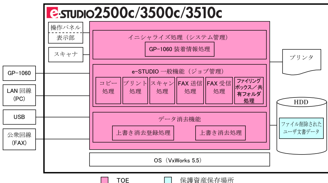
図1-2 通常モード時の構成
