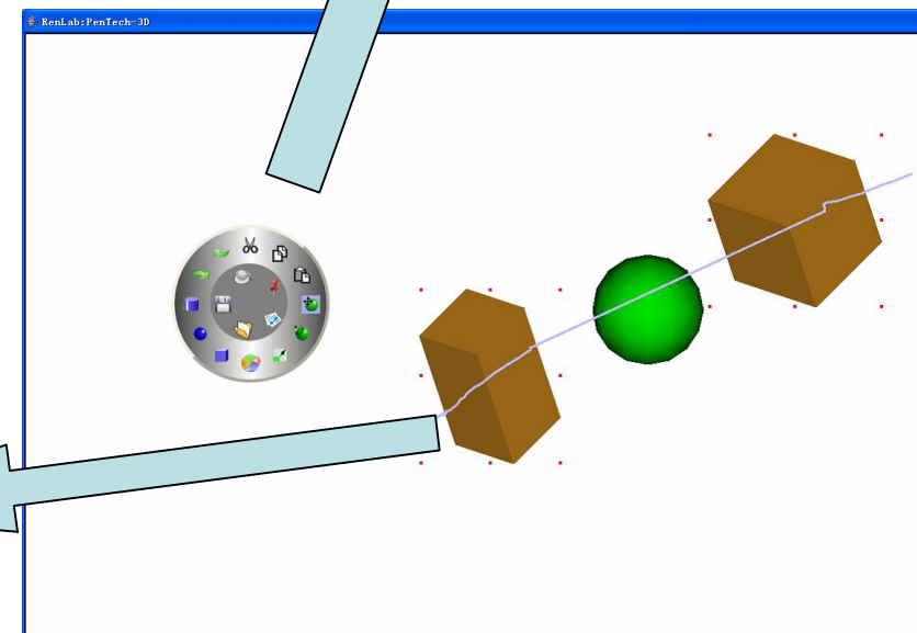
Pie-menu
