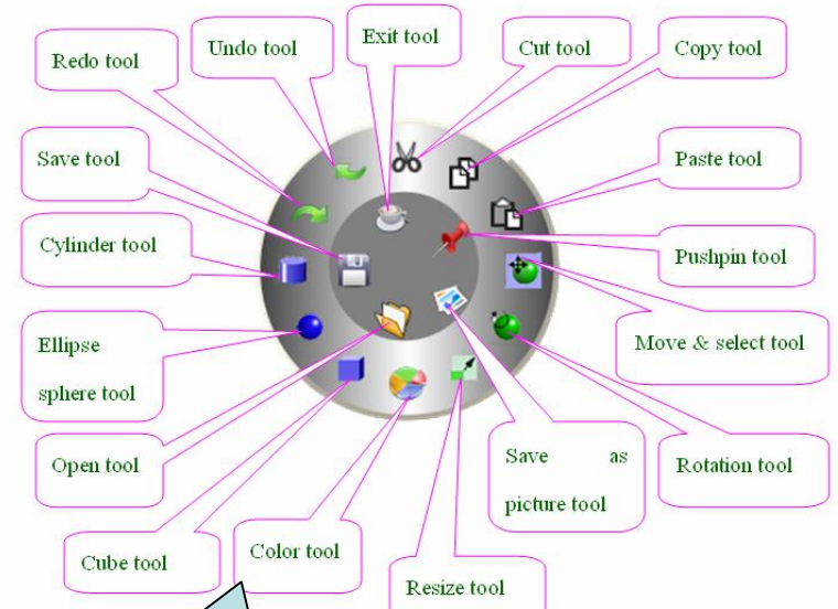
Pie-menu
