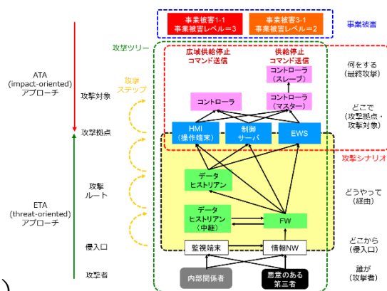
【事業被害、攻撃シナリオ、攻撃ツリーの関係】
