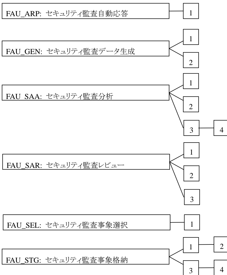
図7 FAU:セキュリティ監査クラスのコンポーネント構成
