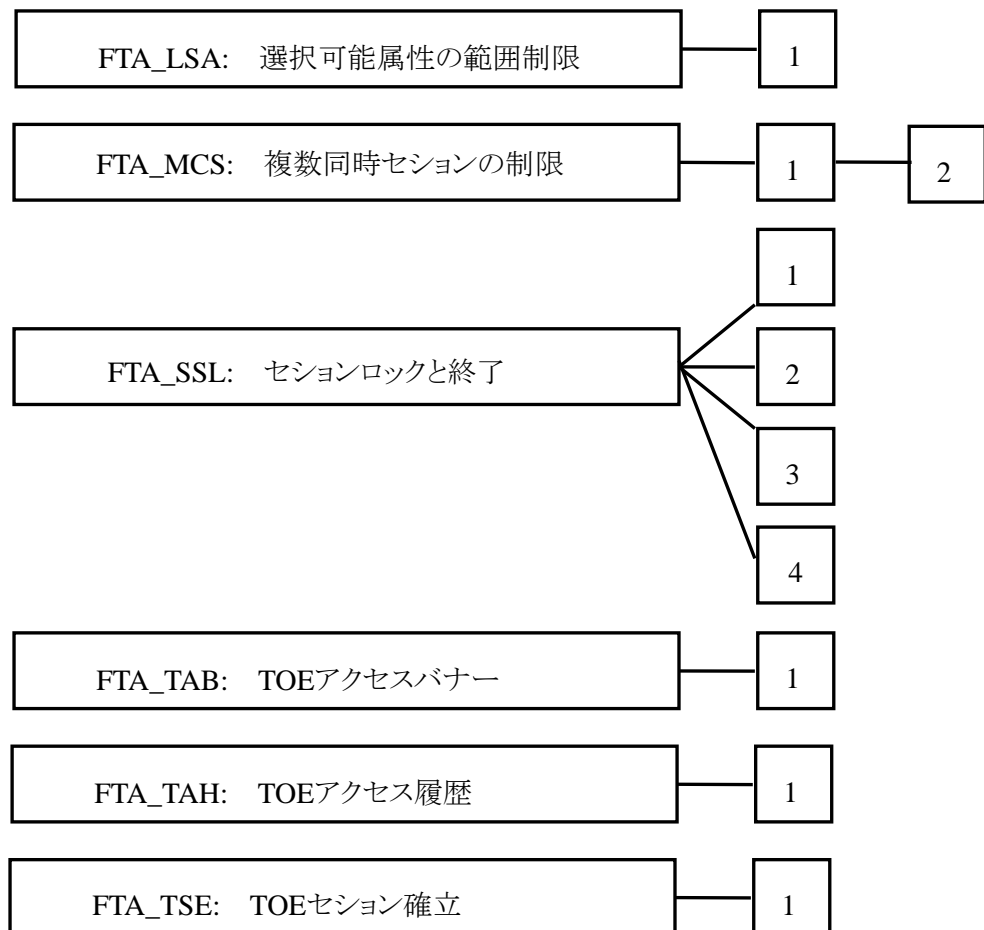
図 30 FTA: TOE アクセスクラスのコンポーネント構成
