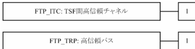
図 17 FTP: 高信頼パス/チャンネルクラスのコンポーネント構成
