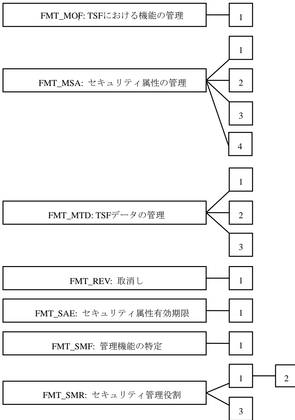
図 12 FMT: セキュリティ管理クラスのコンポーネント構成
