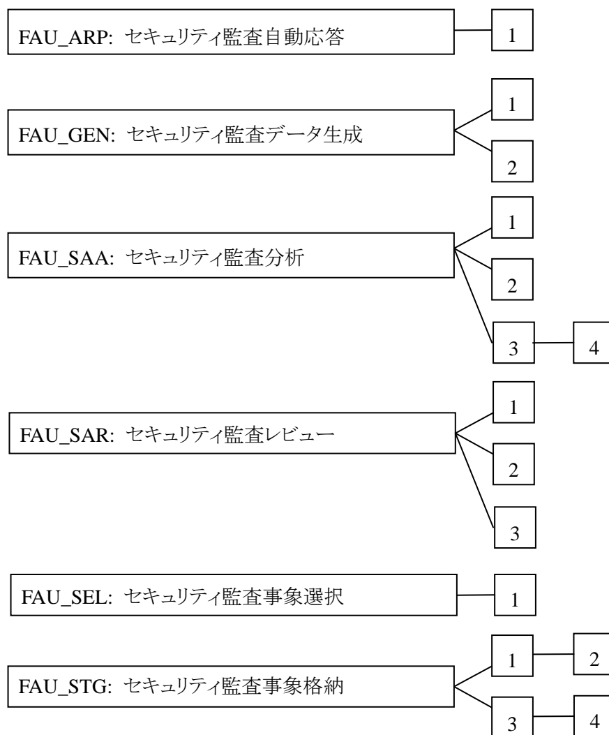
図 21 FAU: セキュリティ監査クラスのコンポーネント構成
