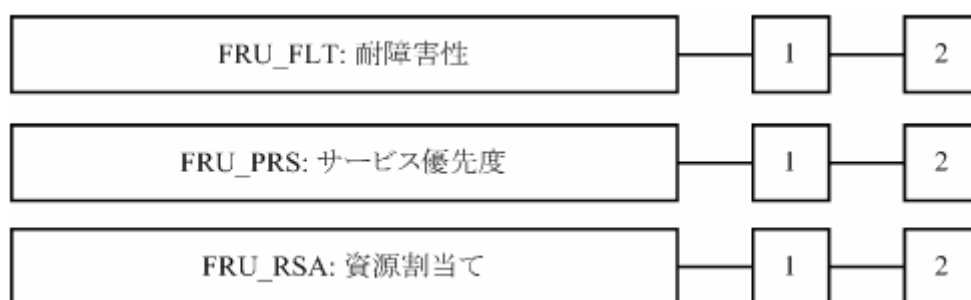
図 29 FRU: 資源利用クラスのコンポーネント構成
