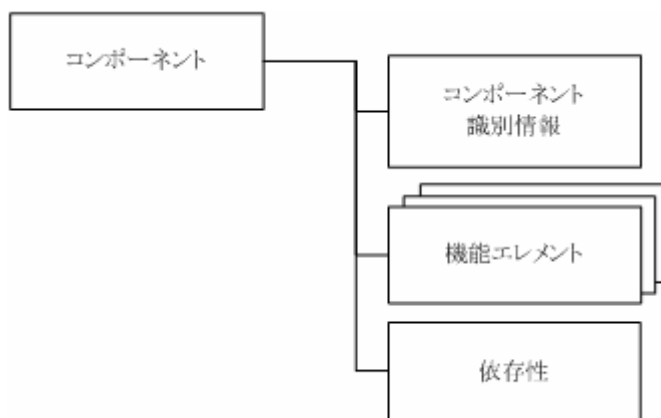
図5 機能コンポーネント構造
