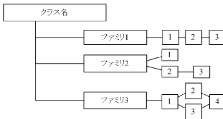
図 6 サンプルクラスのコンポーネント構成図
