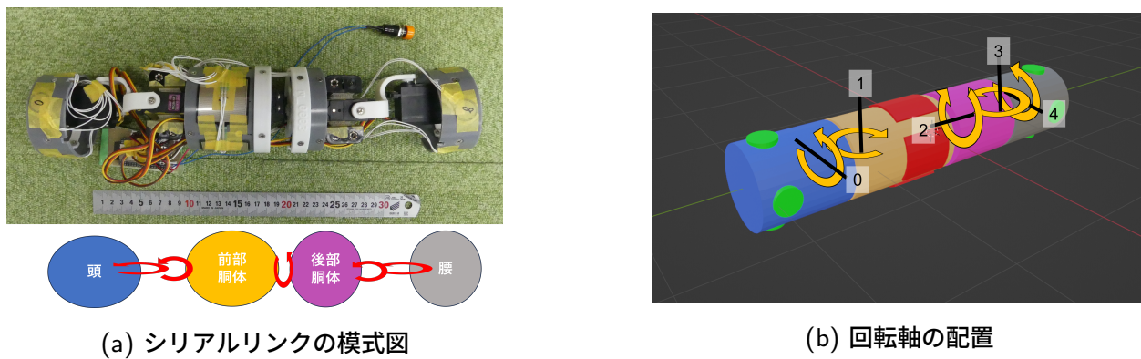
Fig.2: 内部骨格のシリアルリンクの構造と回転軸の配置
